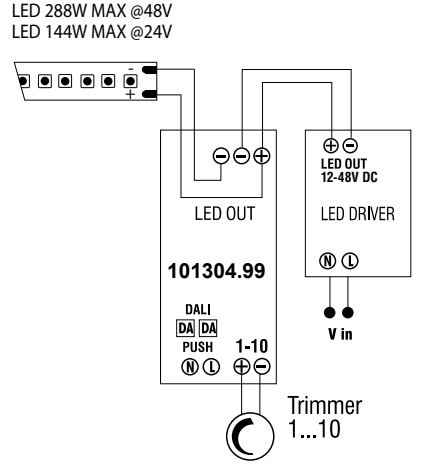
Schema di collegamento trimmer 1...10V, 0...10V 1/10V, 0/10V wiring diagram
