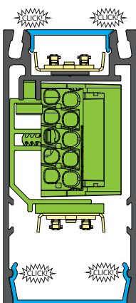
VISTA FRONTALE HERO MINI B MODULO LED E SCHERMO OPALE Hero mini B front view LED module and opal screen
