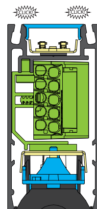
VISTA FRONTALE HERO MINI B MODULO LED MICRO OTTICHE Hero mini front view Micro optics LED module
