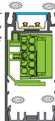
VISTA FRONTALE HERO MINI B MODULO SPOT LED KLIMT Hero mini front view Klimt spot LED module
